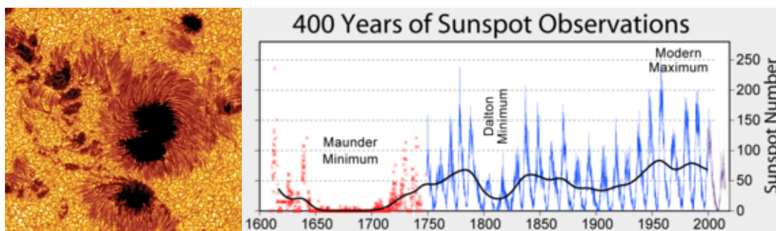
Figuur 1. Het verloop van 400 jaar metingen van zonnevlekken.
